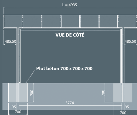
Modèle OXYGEN® toit asymétrique 1 hauteur.
